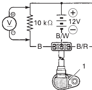
1. Sensor de velocidad
